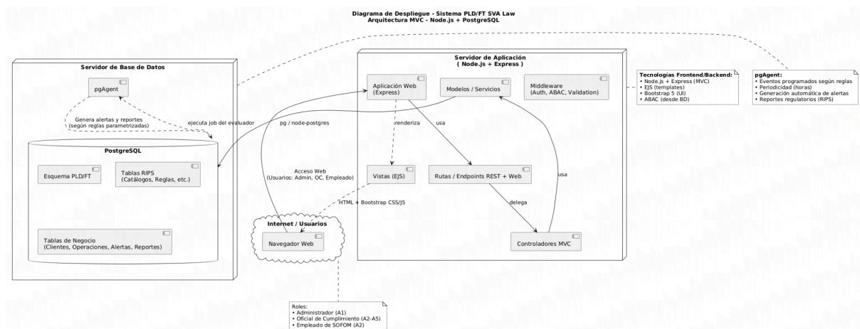
Figura 1. Diagrama de Despliegue entre los distintos actores y componentes del sistema
